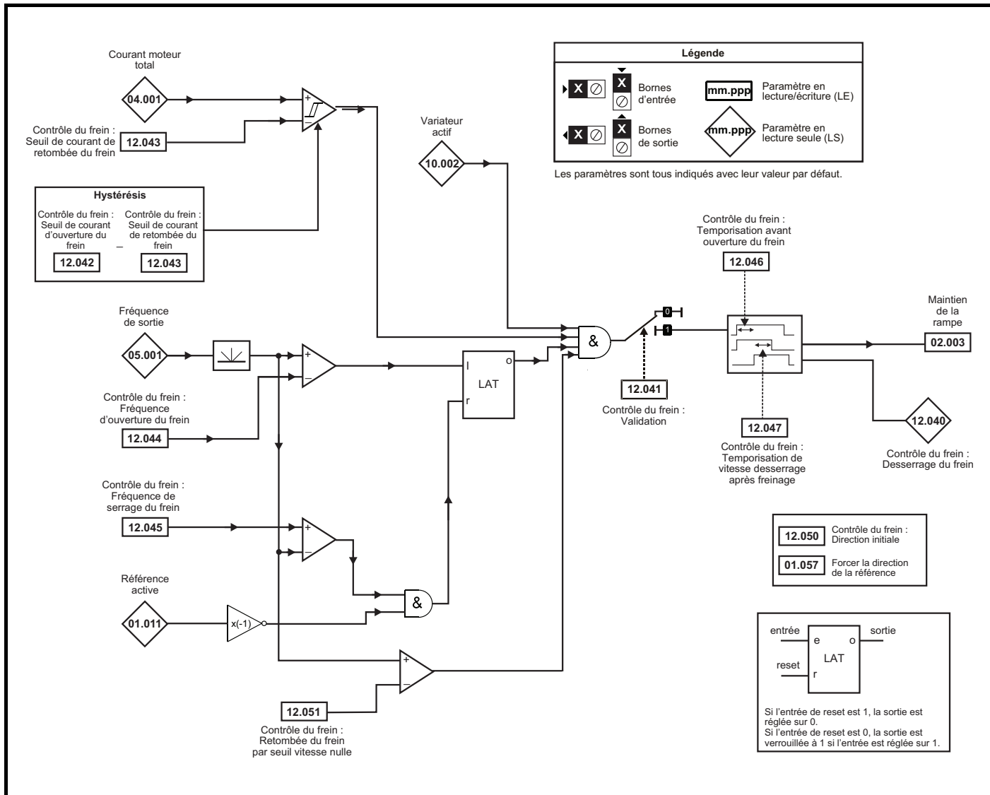
Figure 11-21 Fonction de freinage en boucle ouverte
