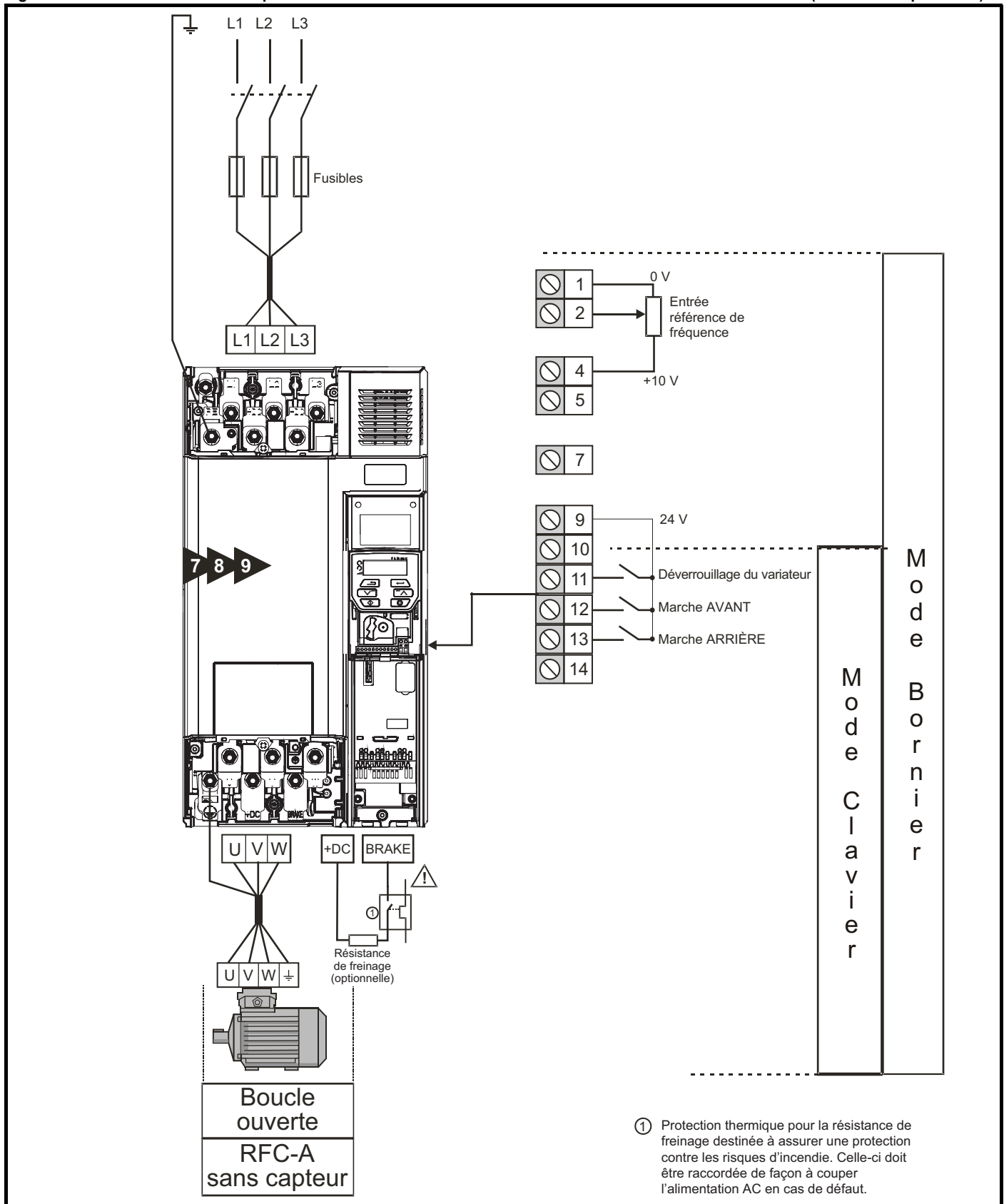
Figure 7-4 Connexions minimales pour la mise en marche du moteur dans tous les modes de fonctionnement (tailles 7 et supérieures)
