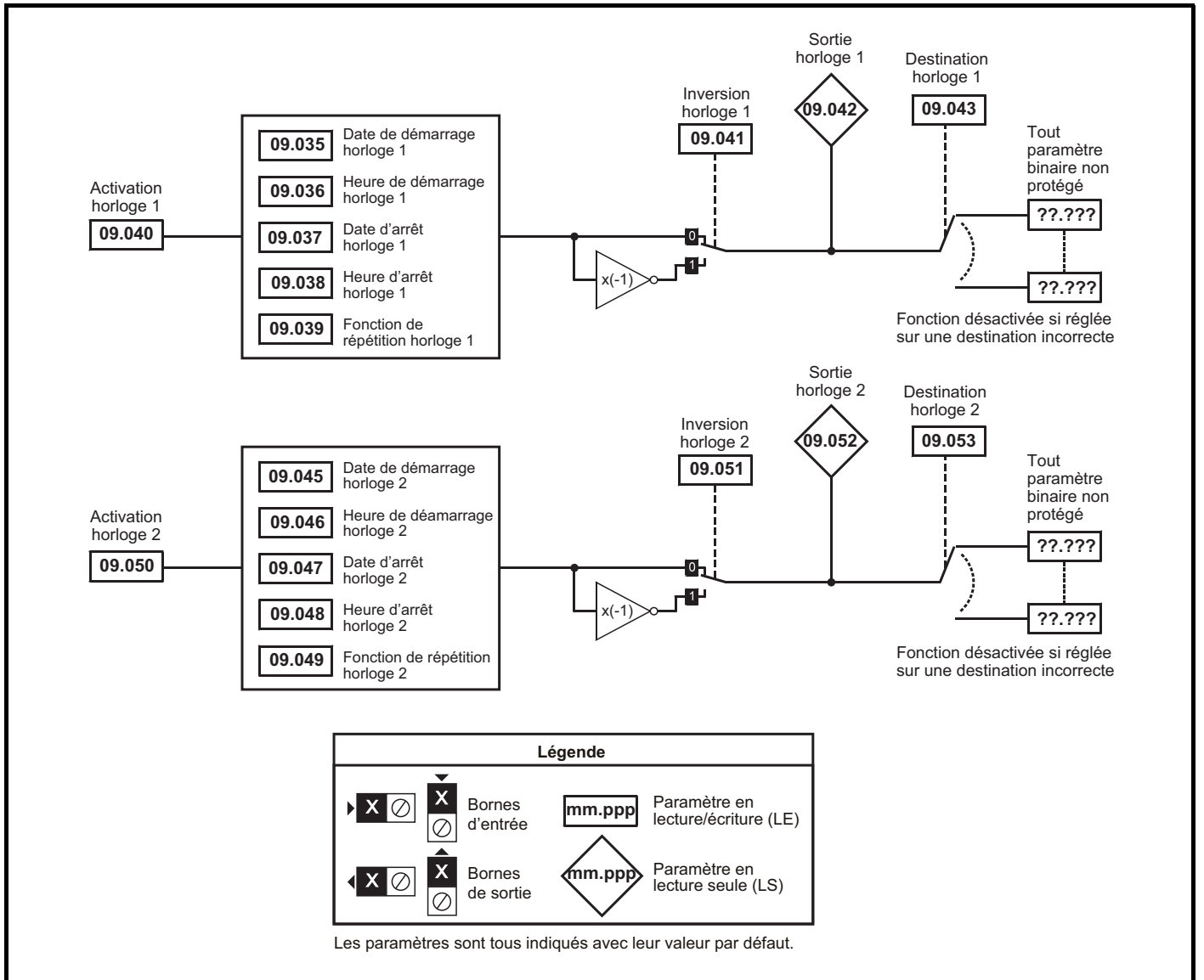
Figure 11-18 Schéma logique du menu 9 : Horloges
