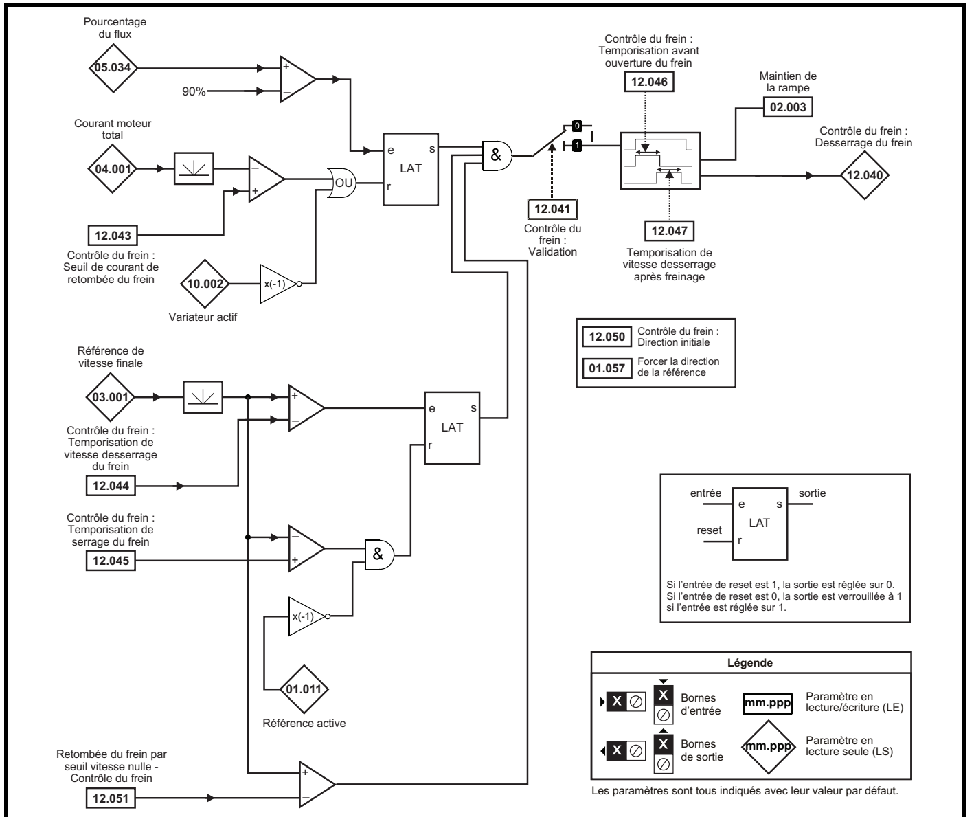
Figure 11-23 Fonction de freinage RFC-A
