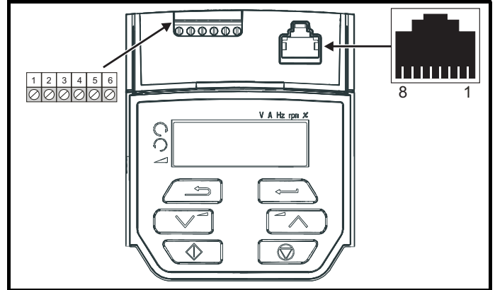
Figure 4-2 Emplacement de l'option AI-485 Adaptor
