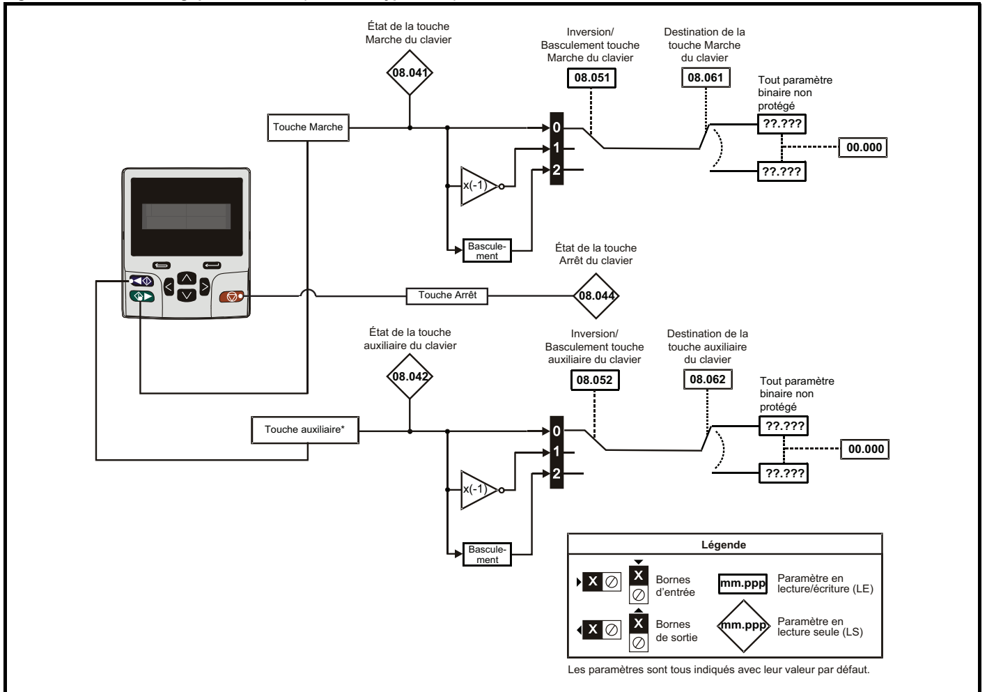
Figure 11-15 Schéma logique du menu 8 (Remote Keypad RTC)
