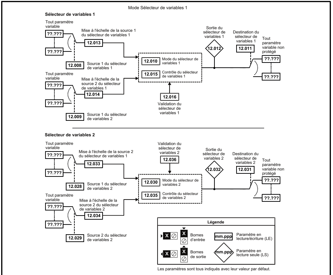
Figure 11-20 Schéma logique du menu 12 (suite)
