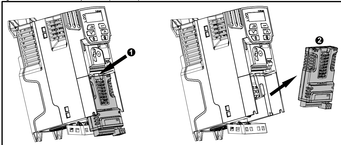
Figure 3-2 Retrait du module optionnel SI (tailles 2 à 4)
