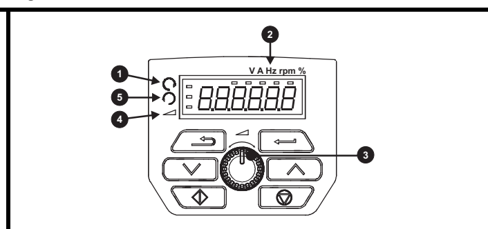
Figure 2-3 Fonction du clavier de l'Unidrive M201
