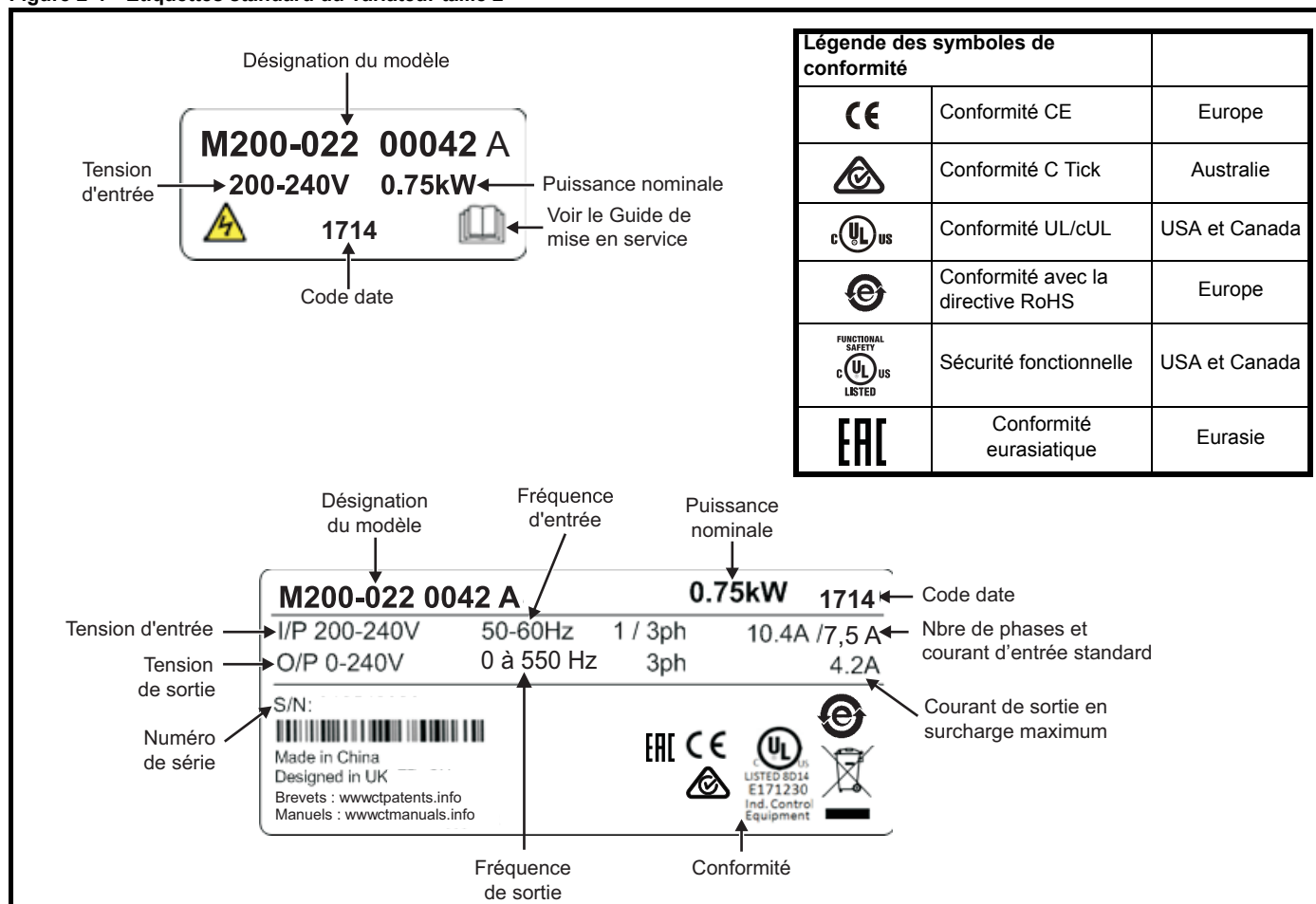
Figure 2-4 Étiquettes standard du variateur taille 2
