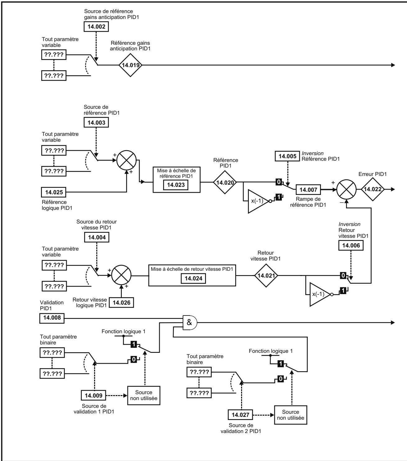
Figure 11-24 Schéma logique du menu 14
