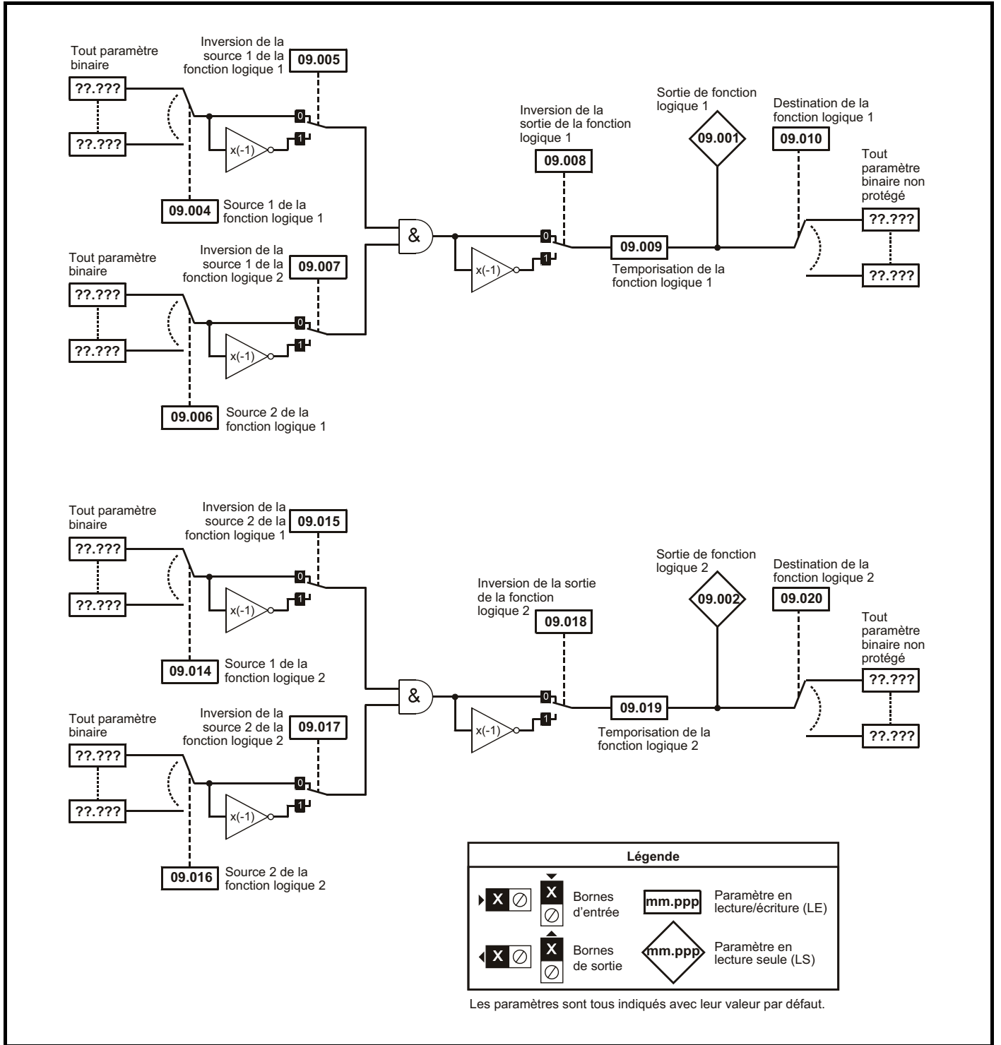
Figure 11-16 Schéma logique du menu 9 : Fonctions logiques
