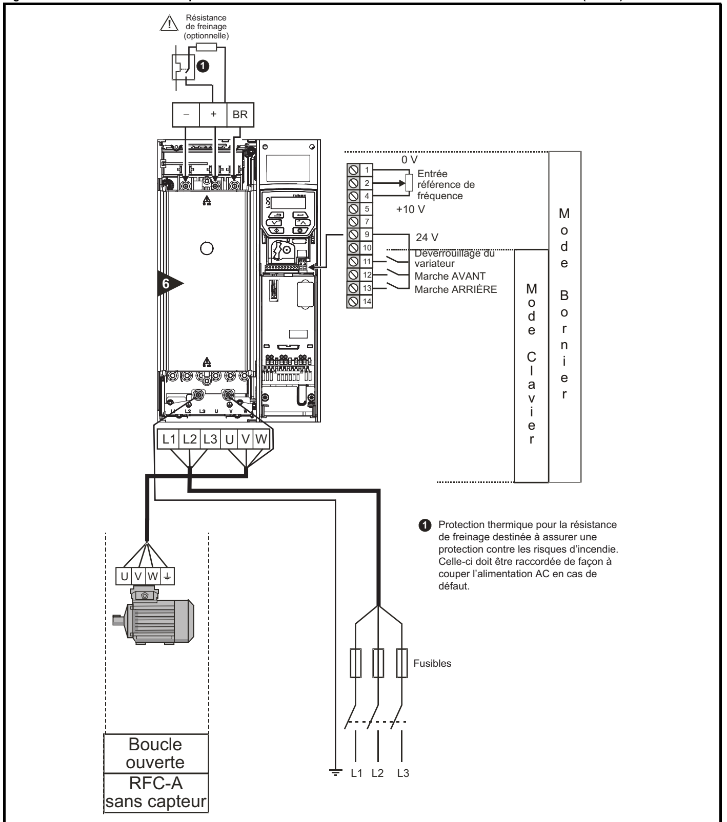
Figure 7-3 Connexions minimales pour la mise en marche du moteur dans tous les modes de fonctionnement (taille 6)
