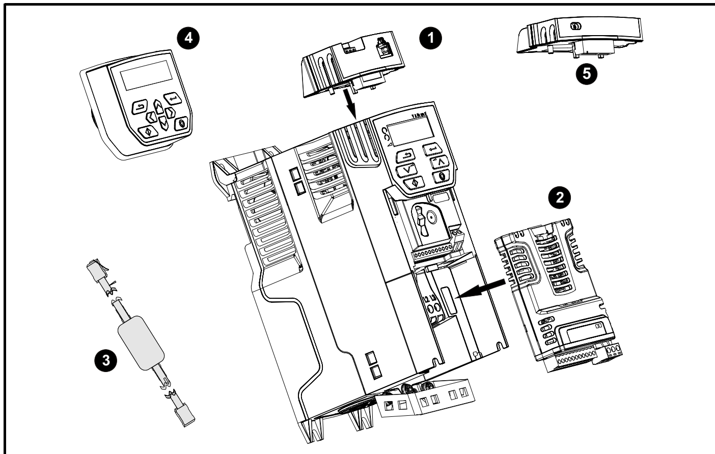
Figure 2-5 Options disponibles avec le variateur
