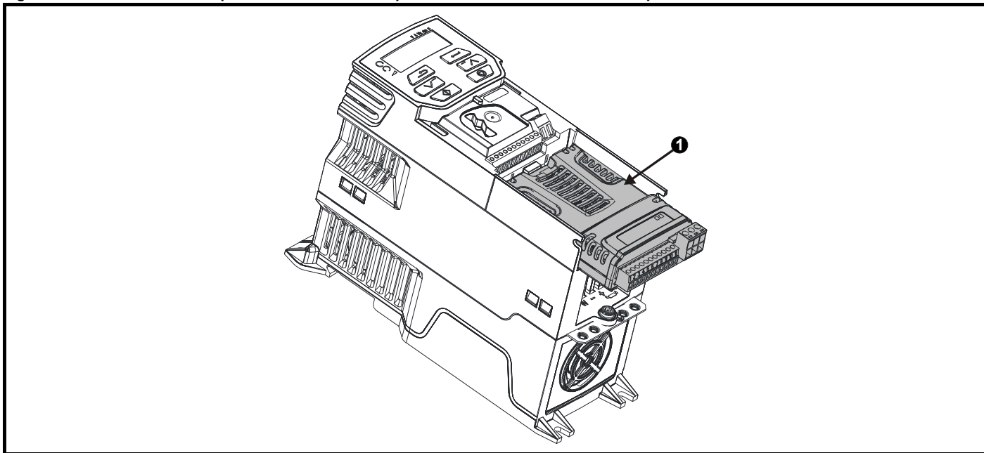
Figure 11-25 Position des emplacements de module optionnel et numéro de menu correspondants
