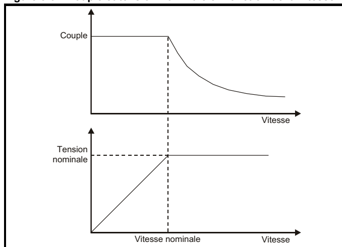
Figure 8-3 Couple et tension nominale en fonction de la vitesse
