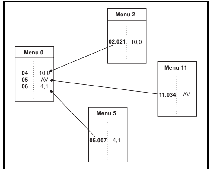
Figure 5-5 Copie de paramètres dans le menu 0
