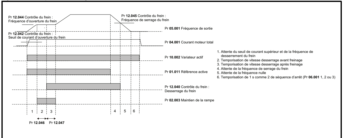
Figure 11-23 Fonction de freinage RFC-A
