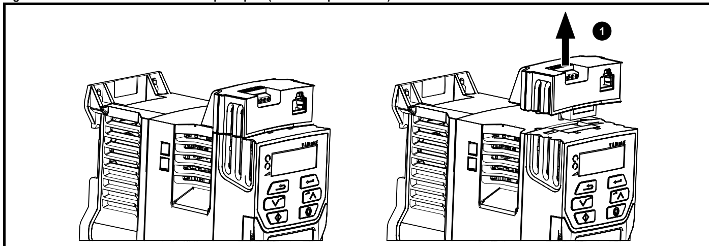
Figure 3-6 Retrait de l'AI-485 / AI-Backup Adaptor (AI-485 Adaptor illustré)
