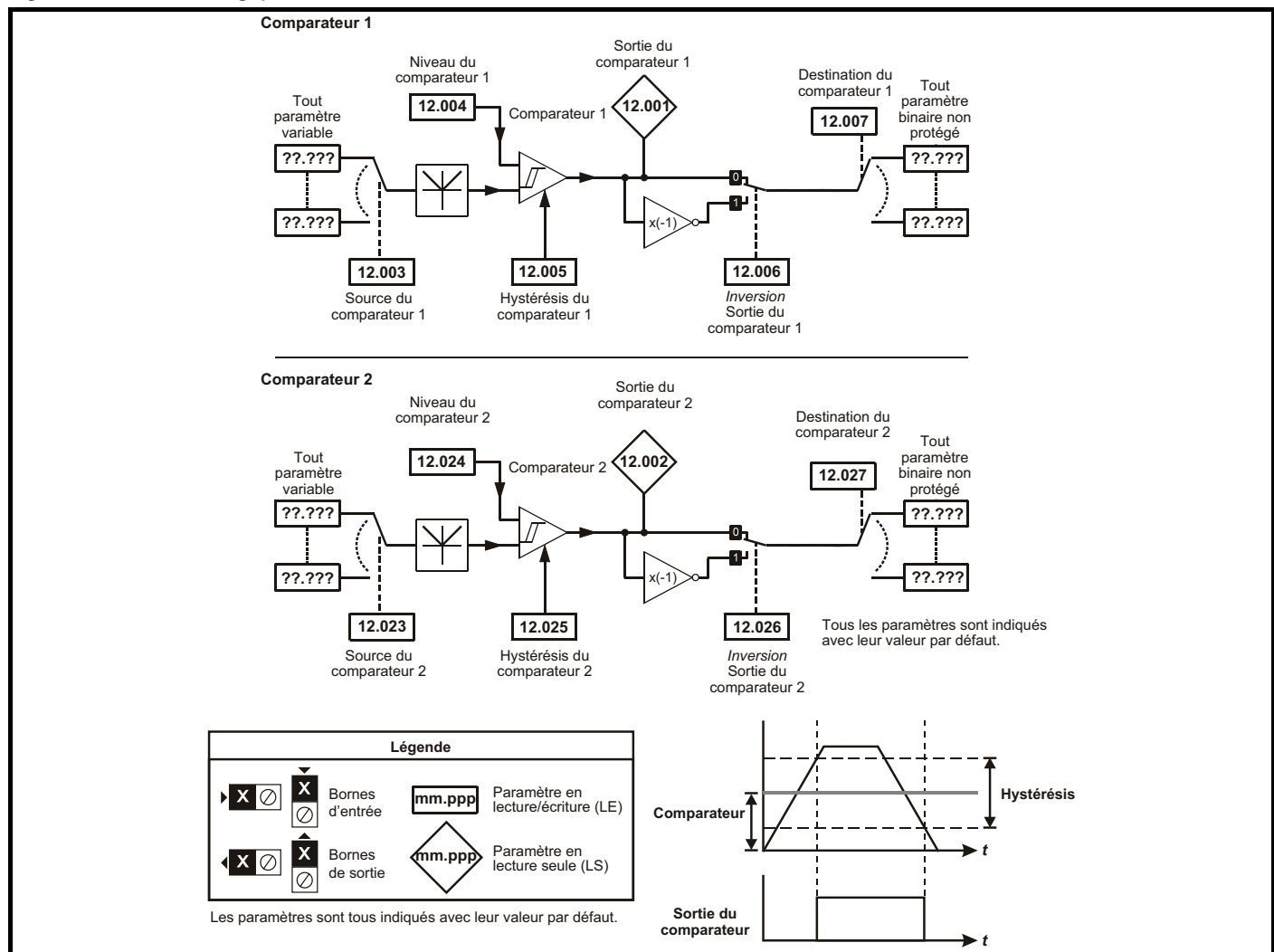
Figure 11-19 Schéma logique du menu 12
