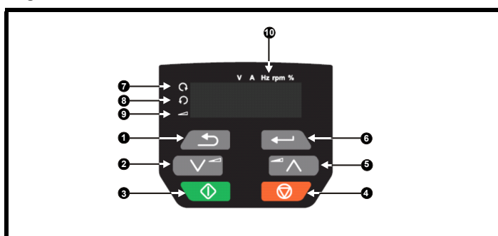
Figure 2-2 Fonction du clavier de l'Unidrive M200
