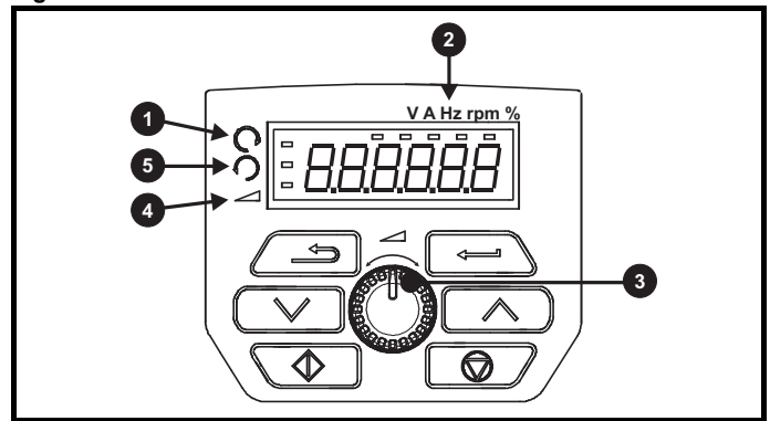
Figure 5-2 Fonction du clavier de l'Unidrive M201
