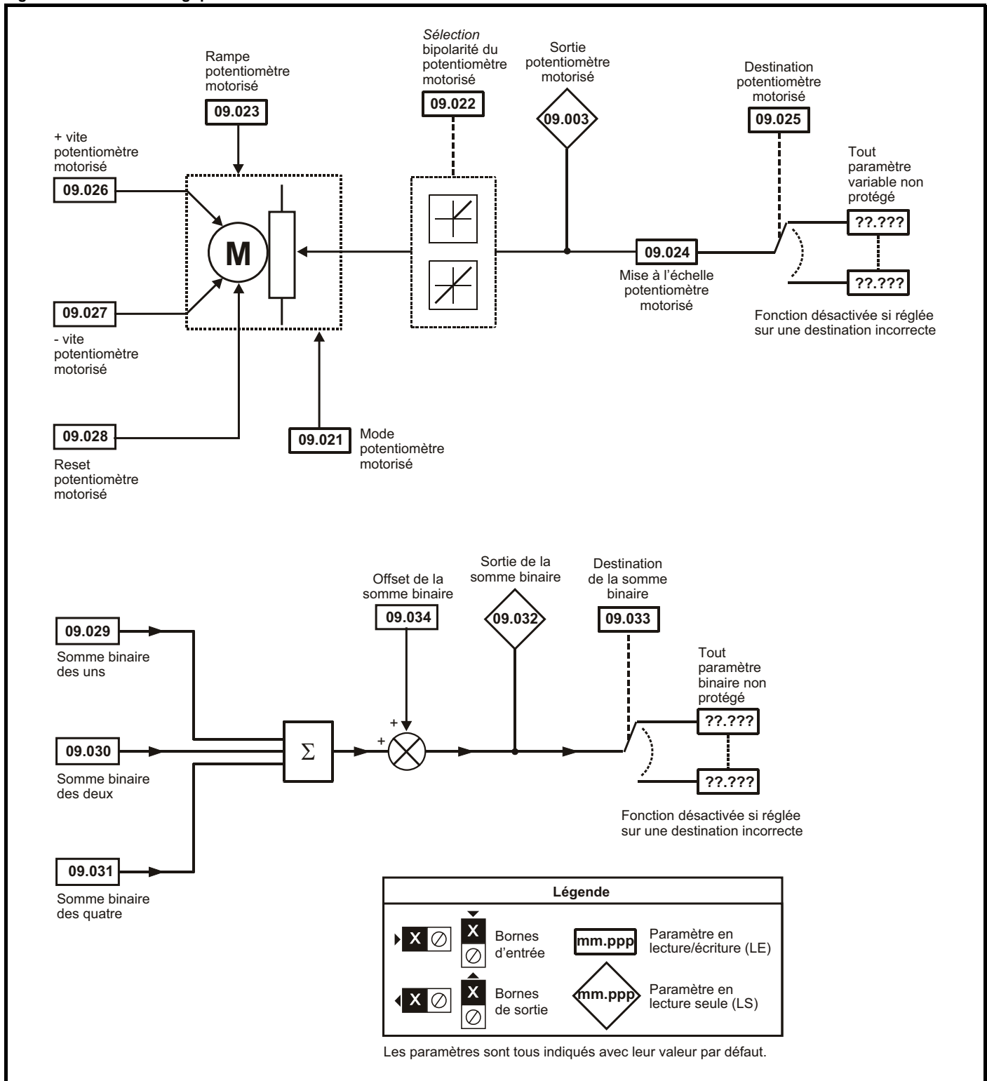
Figure 11-17 Schéma logique du menu 9 : Potentiomètre motorisé et somme binaire
