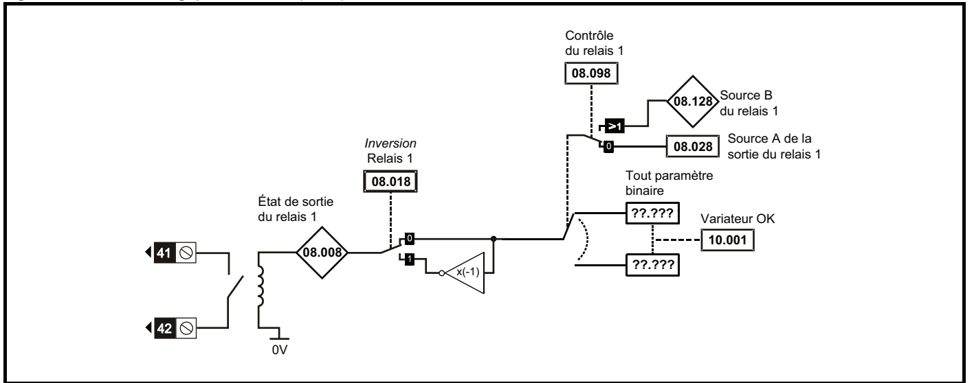
Figure 11-14 Schéma logique du menu 8 (relais)
