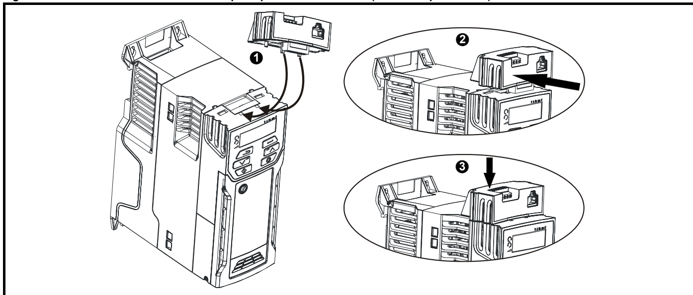
Figure 3-5 Installation de l'AI-485 / AI-Backup Adaptor dans le variateur (AI-485 Adaptor illustré)
